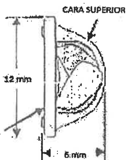
VISTA LATERAL DEL BROCHE
