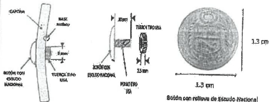
Perno y tuerca tipo USA
